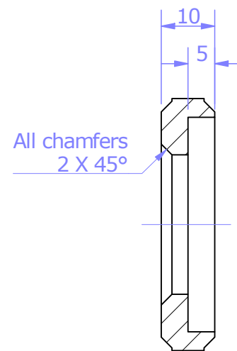
Section D-D
