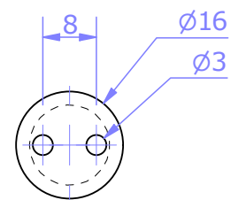
End Elevation
