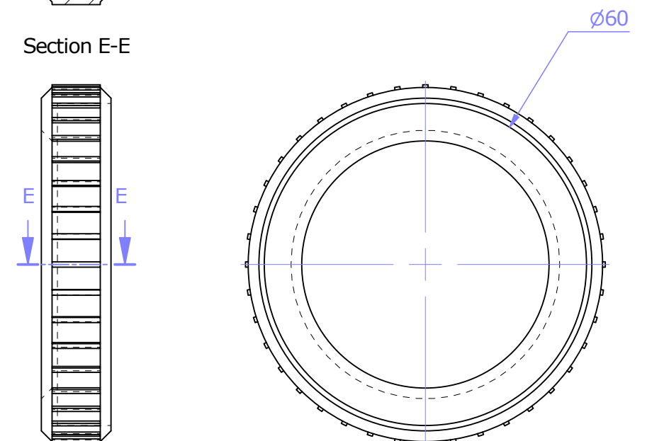
Elevation
