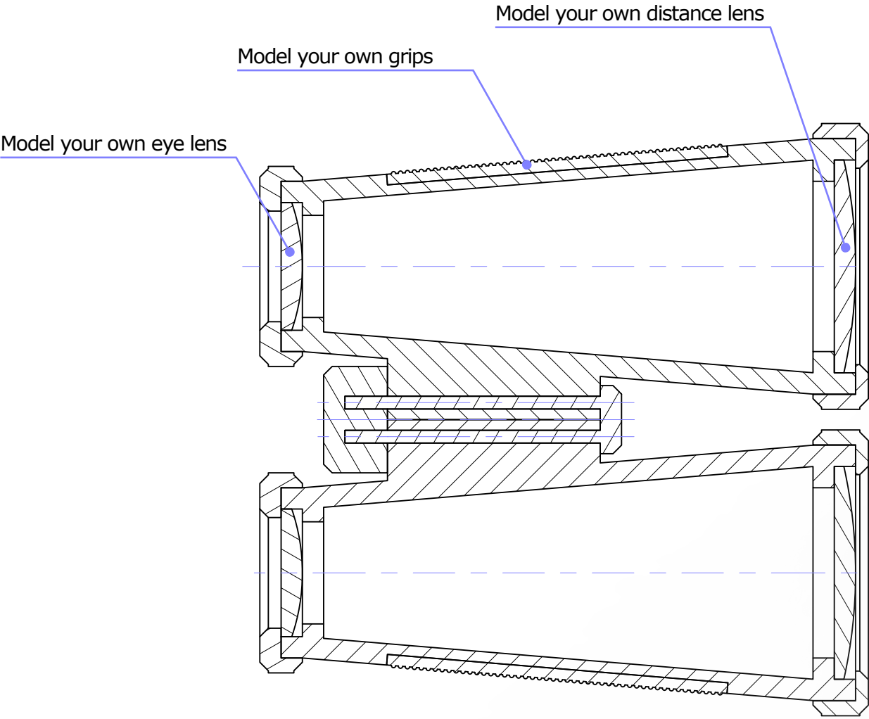
Section A-A
