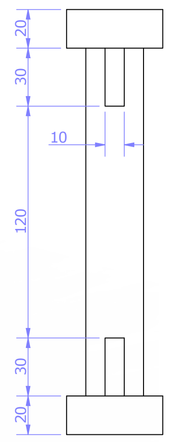
End Elevation
