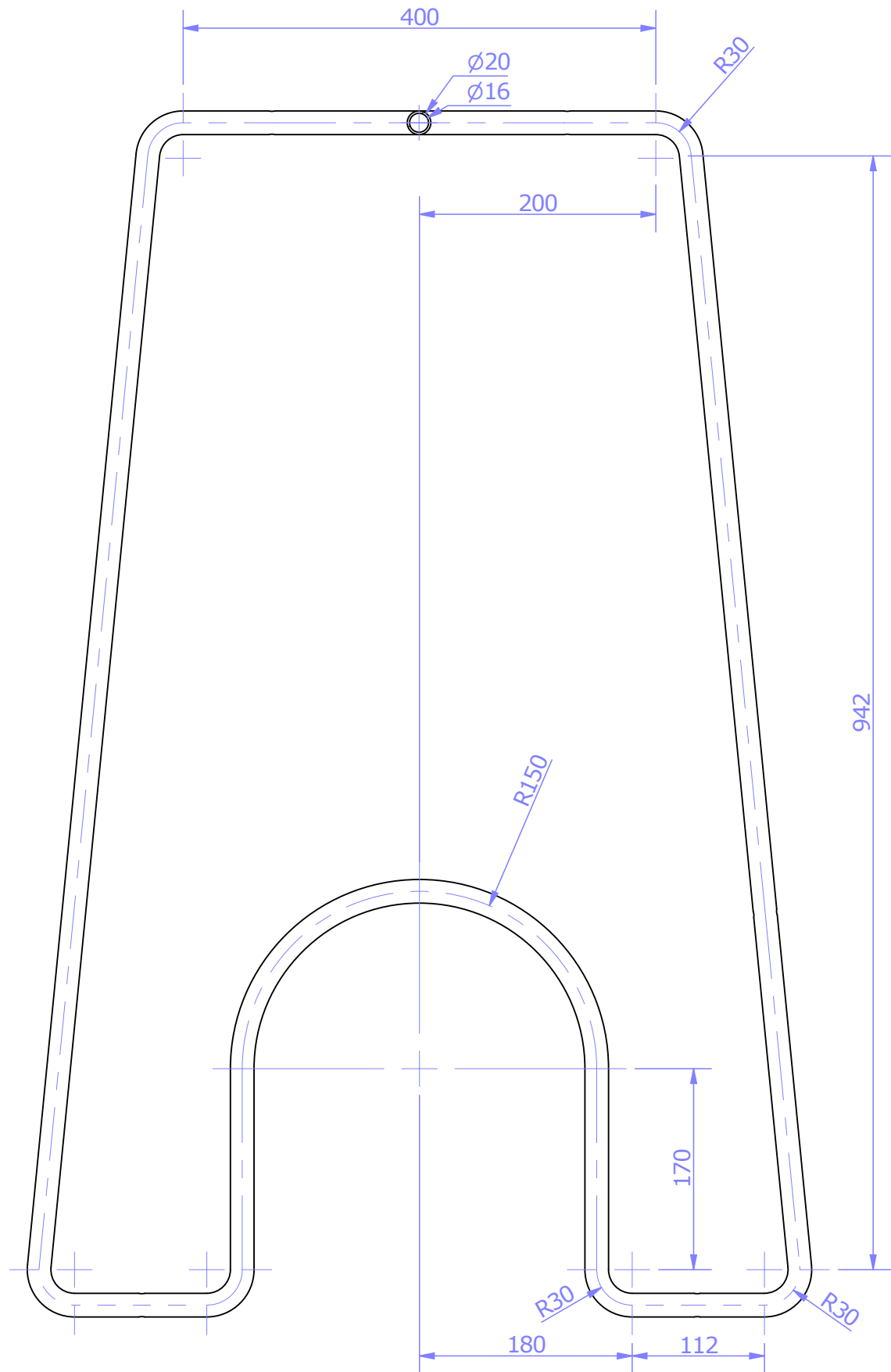
Elevation
