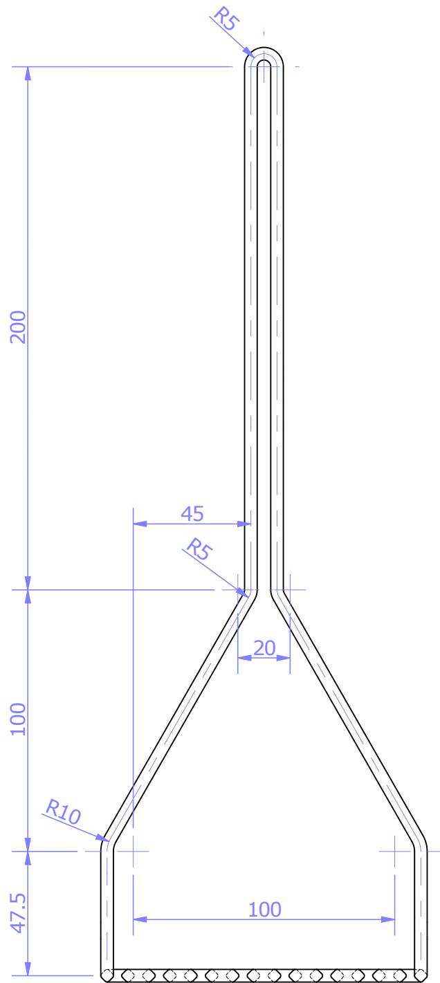
Elevation
