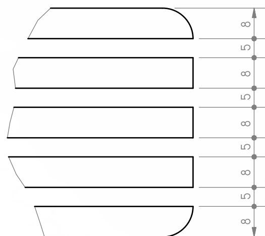
PARTIAL ENLARGEMENT A
