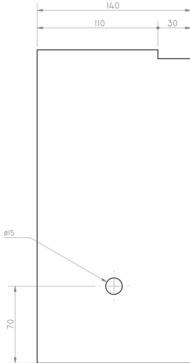
ELEVATION
